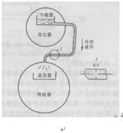
图 5-12 小孔节流装置
