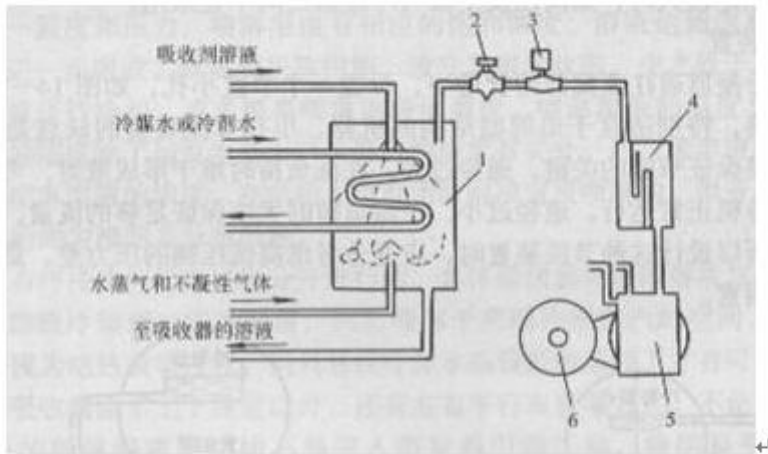
图 5-13 机械真空泵抽气装置 ↓
