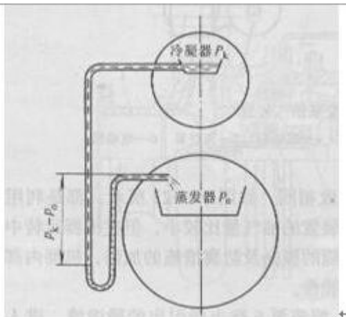
图 5-11 U形管节流装置
